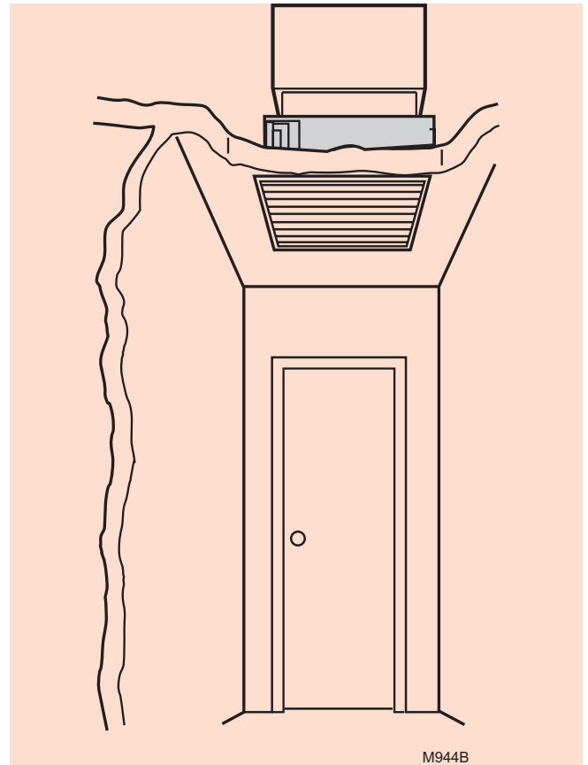
Fig. 6. Installation de ventilation centrale avec épurateur d'air à fibres monté horizontalement dans la gaine de retour centrale.
